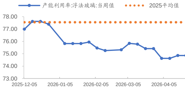
图26 浮法玻璃产能利用率 (%)
